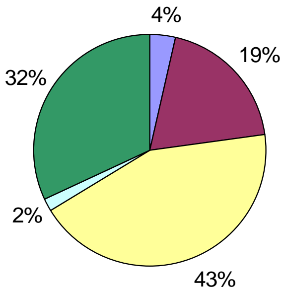
Consommation d'énergie par secteur en France (2008)
