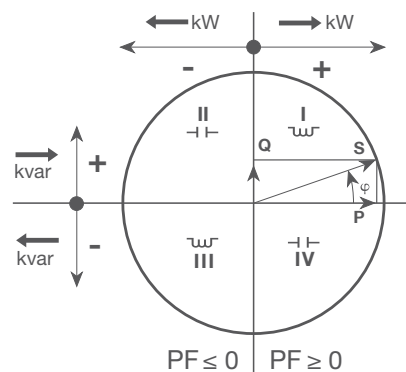
Facteur de puissance Convention selon CEI 62053-23
