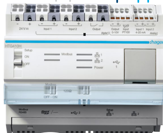
Serveur de surveillance de l'énergie (Modbus Master)
