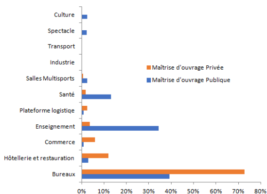
Figure 13 : Répartition des projets tertiaires BBC-Effinergie suivant le type de maîtrise d'ouvrage
