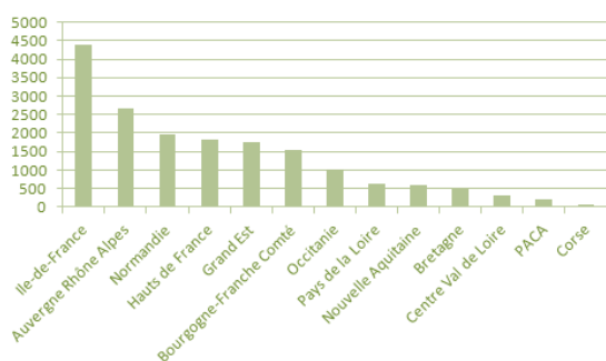
Figure 16 : Nombre de logements rénovés à basse consommation par régions
