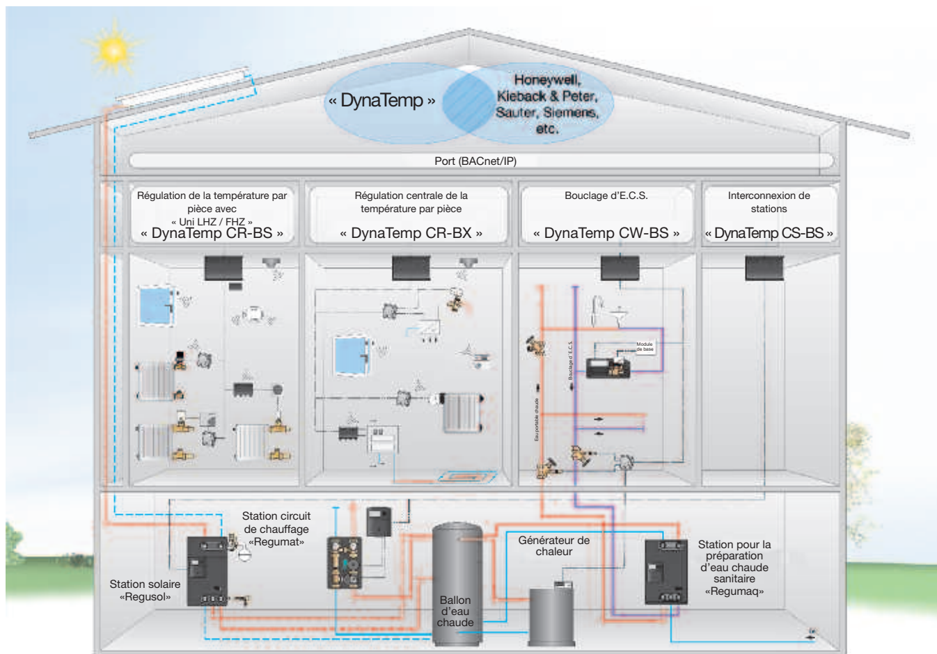
Schéma d'installation
