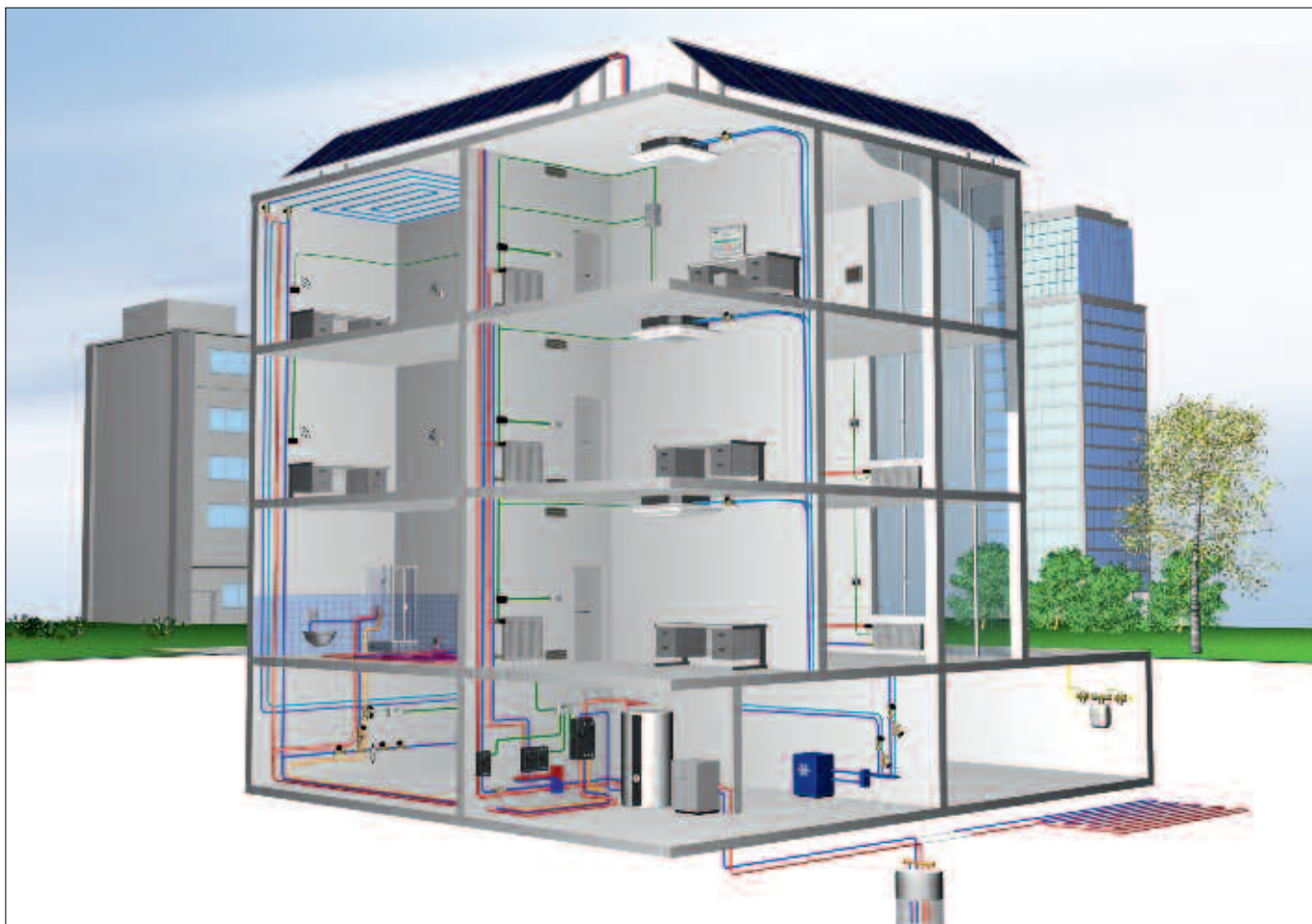
Schéma d'installation
