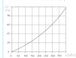
Pertes de charge borne de prise d'air ext. avec filtre G 3 et 40 m de collecteur, titre propre.
