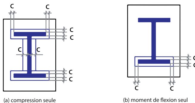
▲ Figure B.5 – Tronçon en Té comprimé
