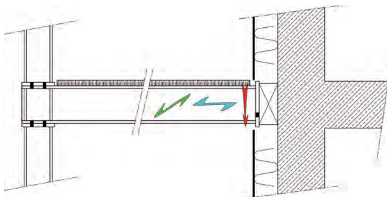
▲ Figure 11 – Exemple de fixation d'un élément en appui avec rupteur thermique
