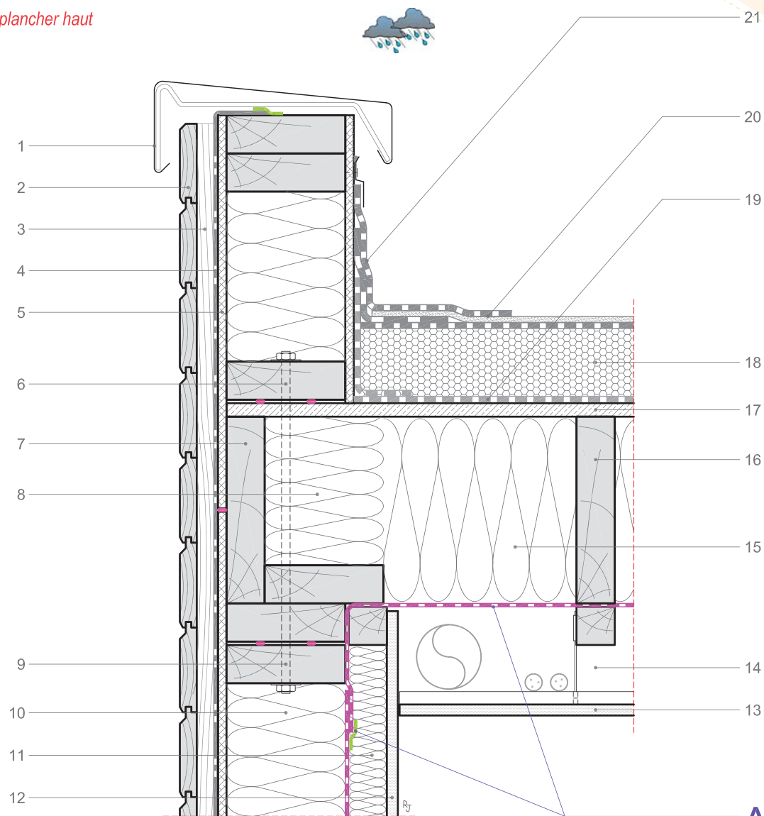
Coupe verticale
