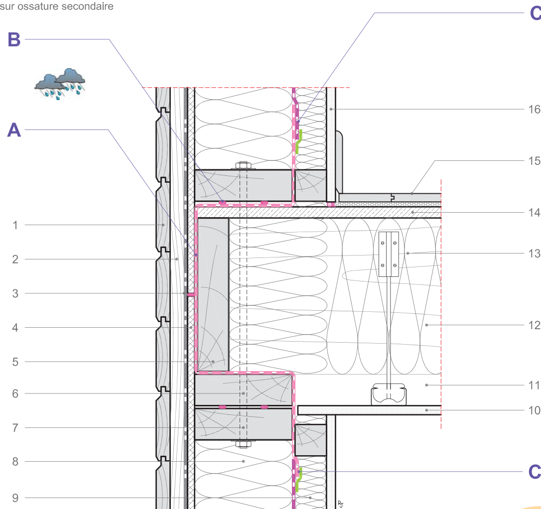
Coupe verticale
