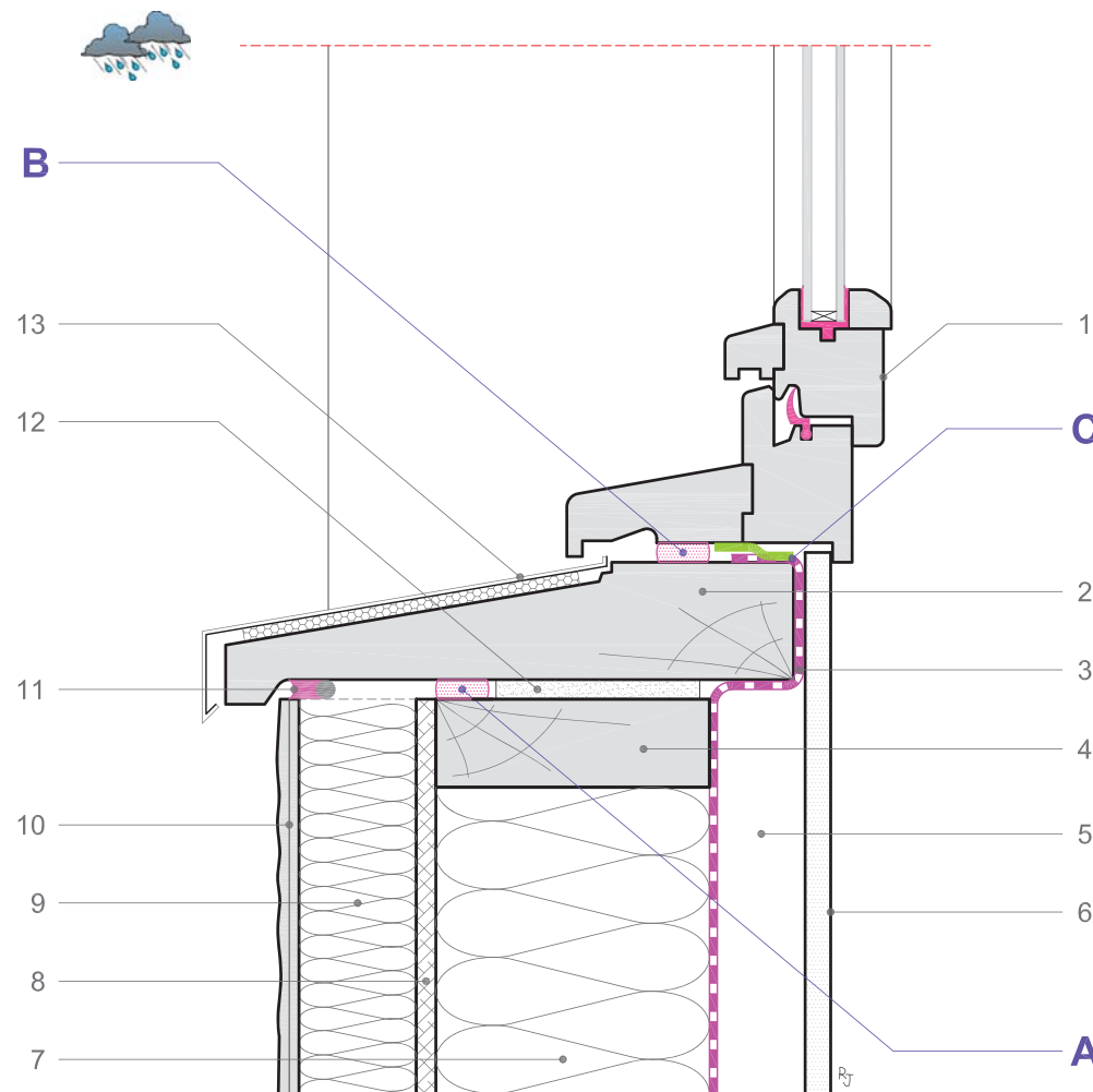
Coupe verticale
