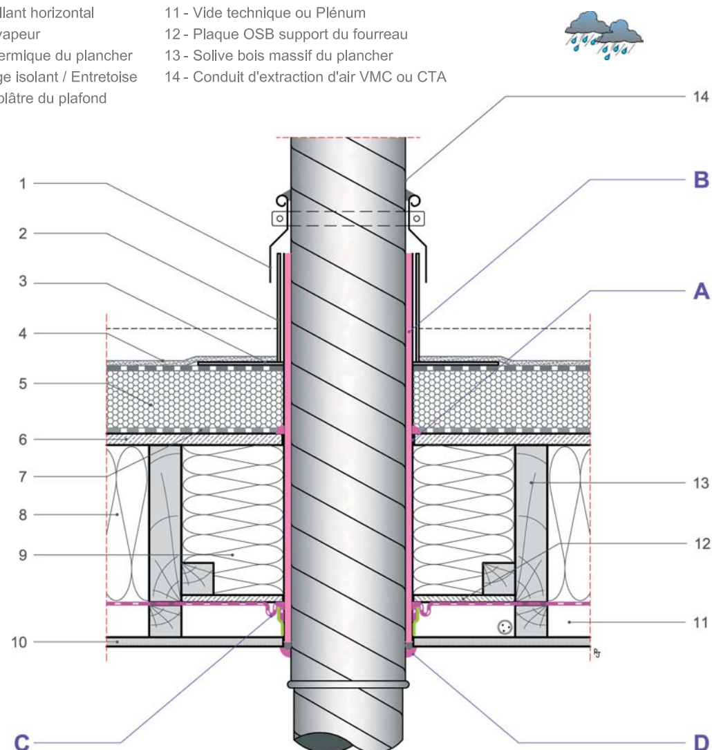
Coupe verticale
