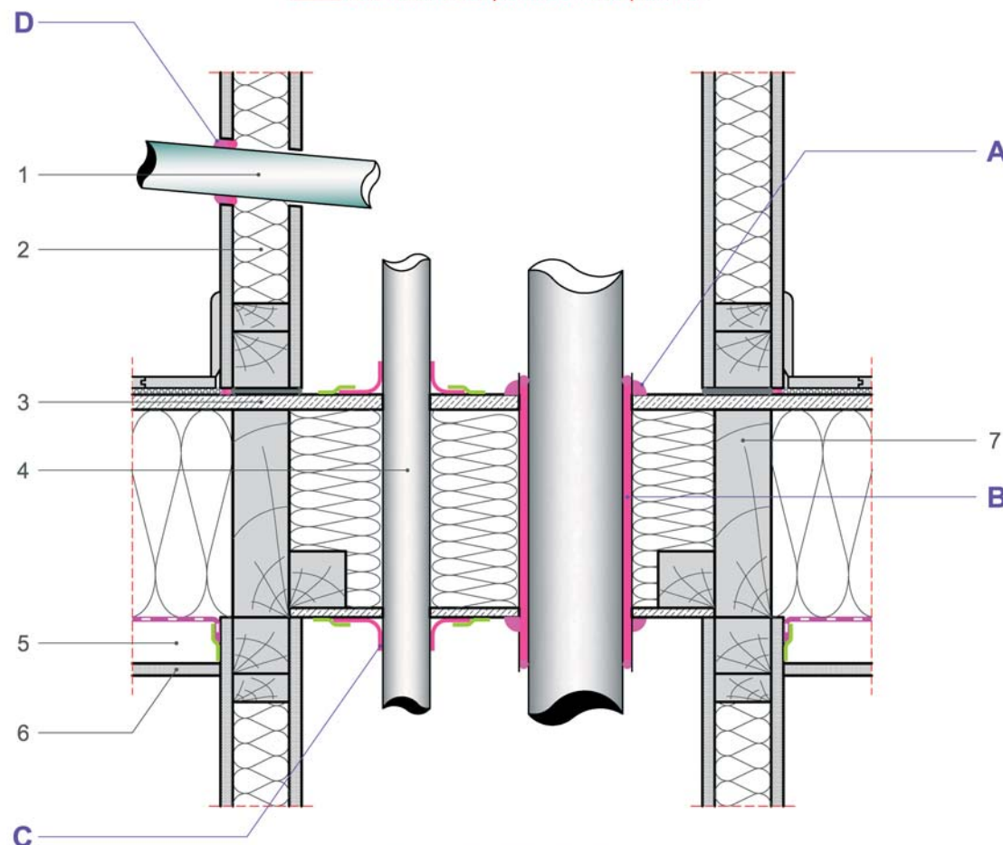
Coupe verticale
