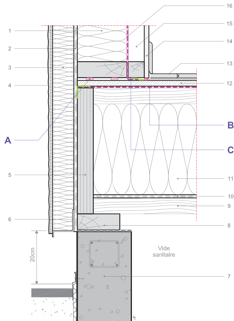
Coupe verticale
