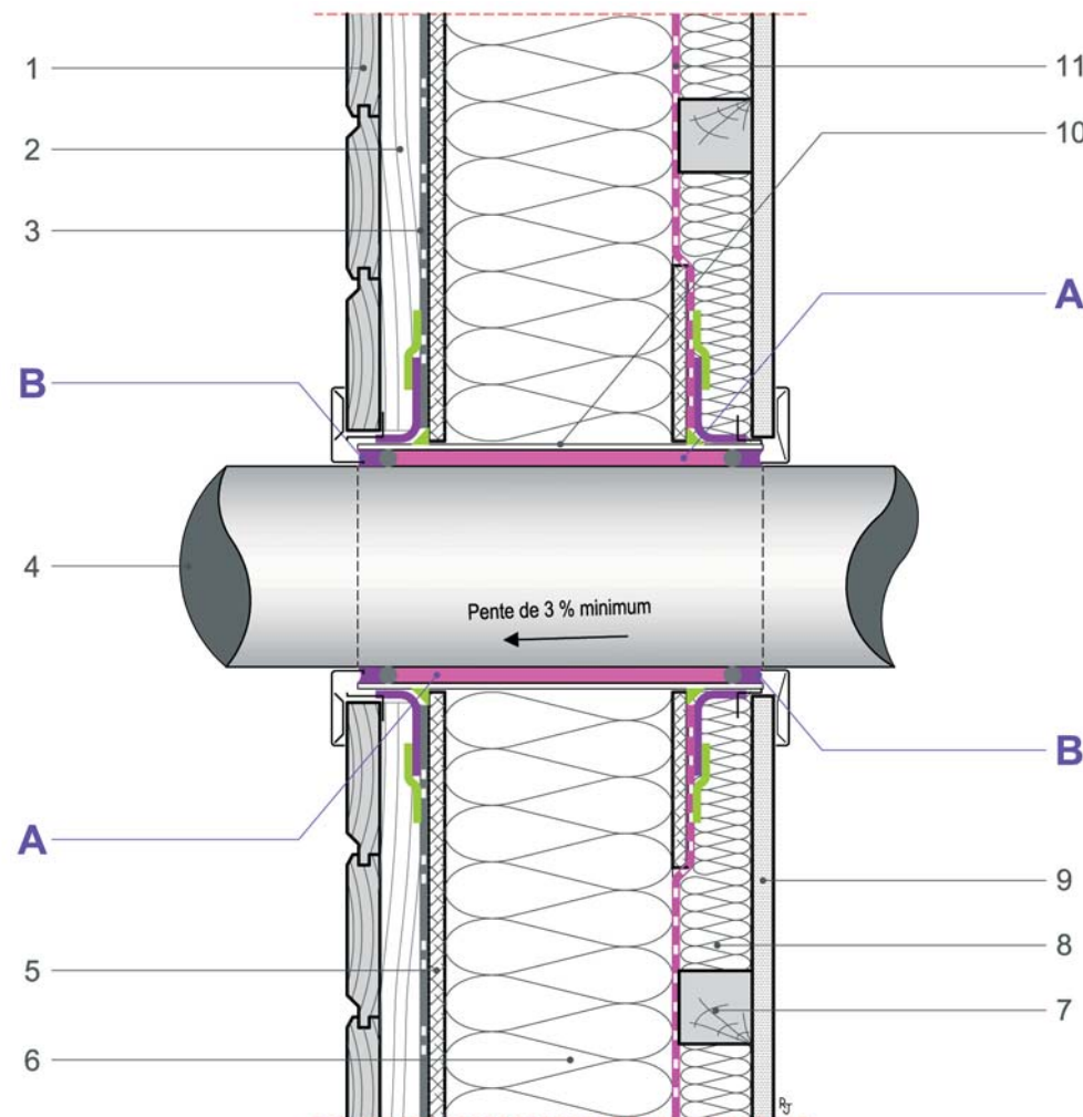
Coupe verticale
