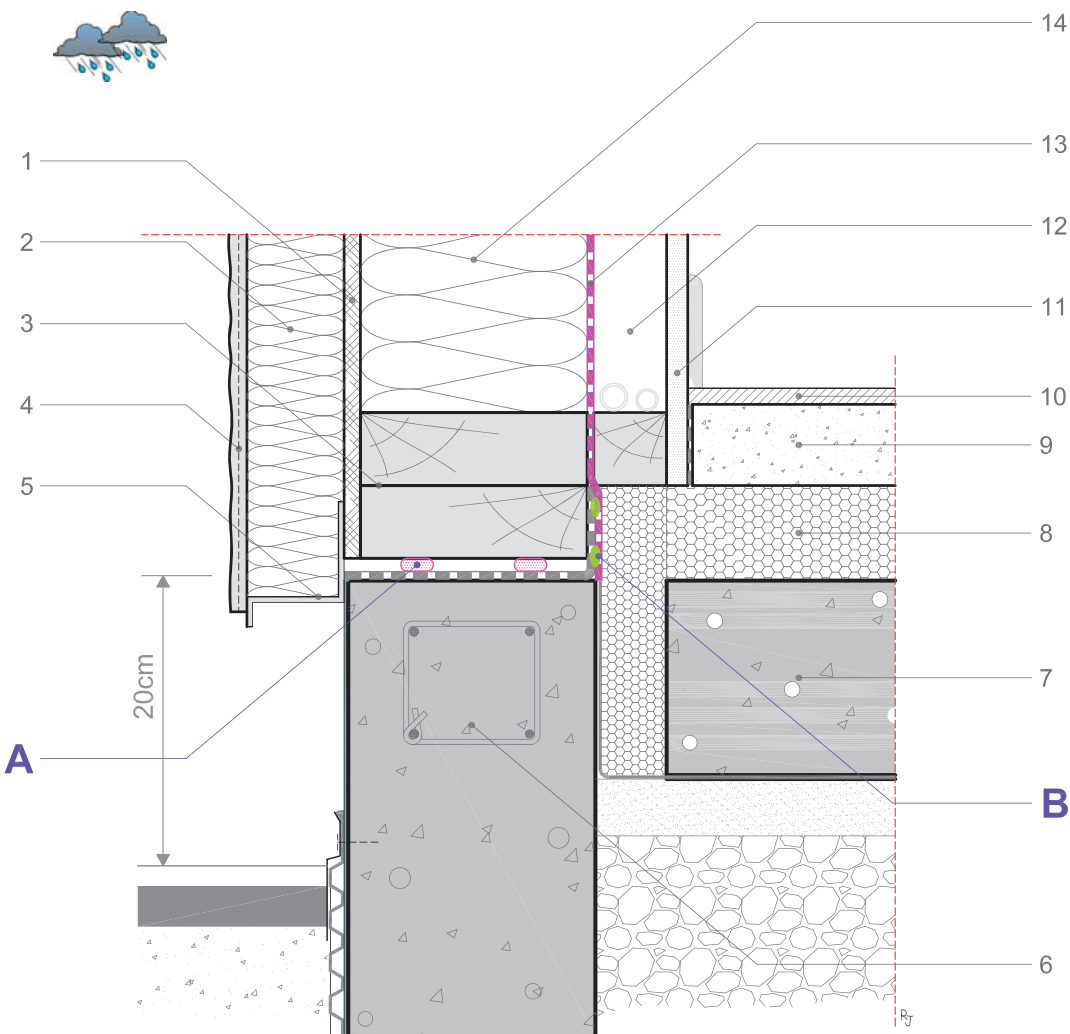
Coupe verticale
