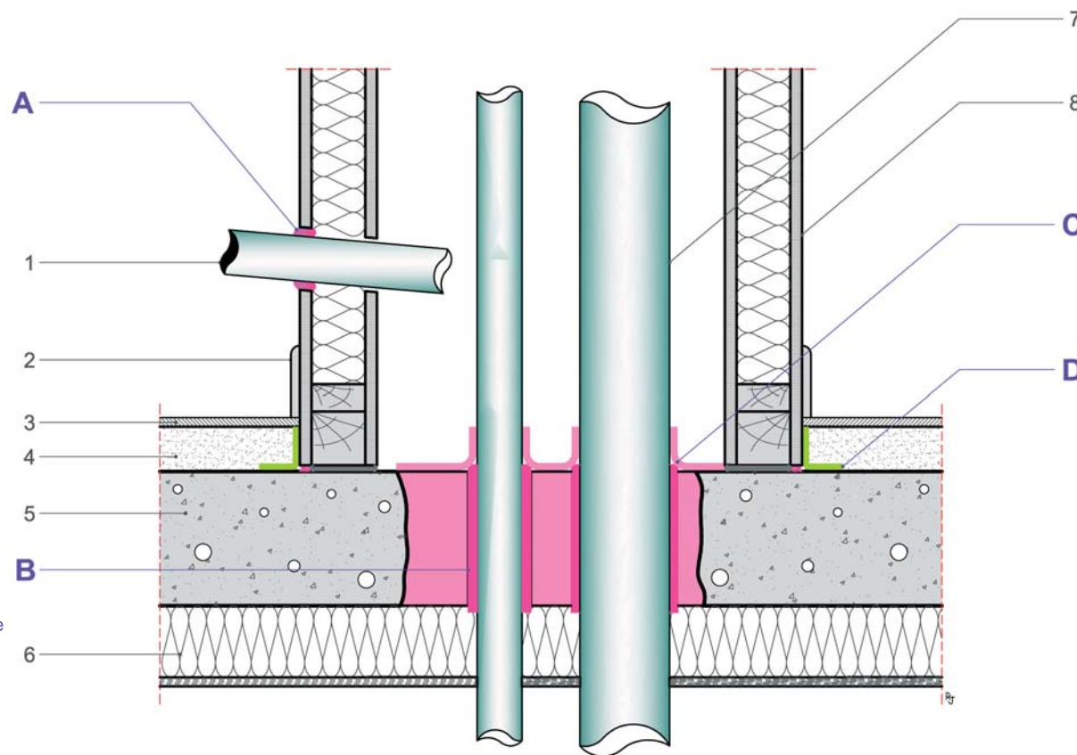
Coupe verticale
