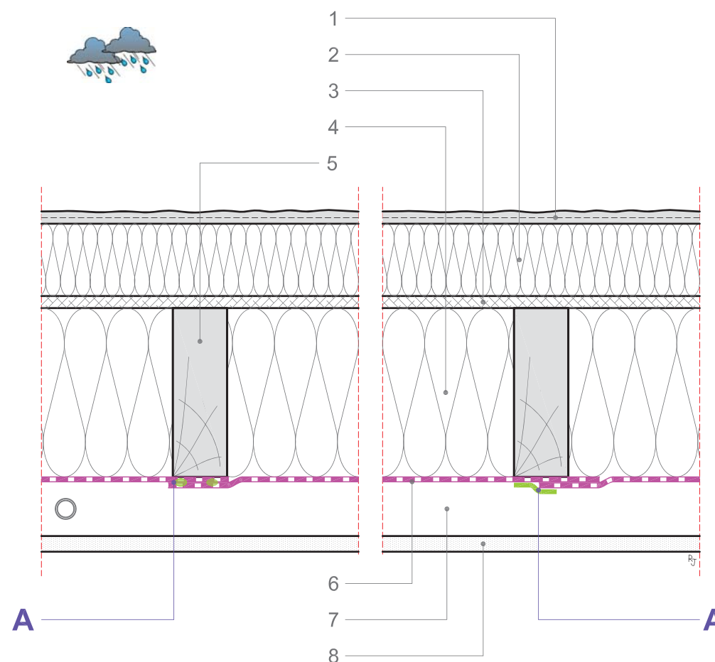
Coupe horizontale
