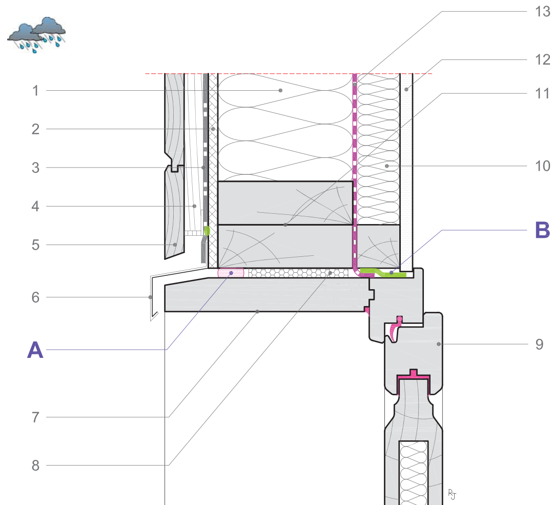
Coupe verticale
