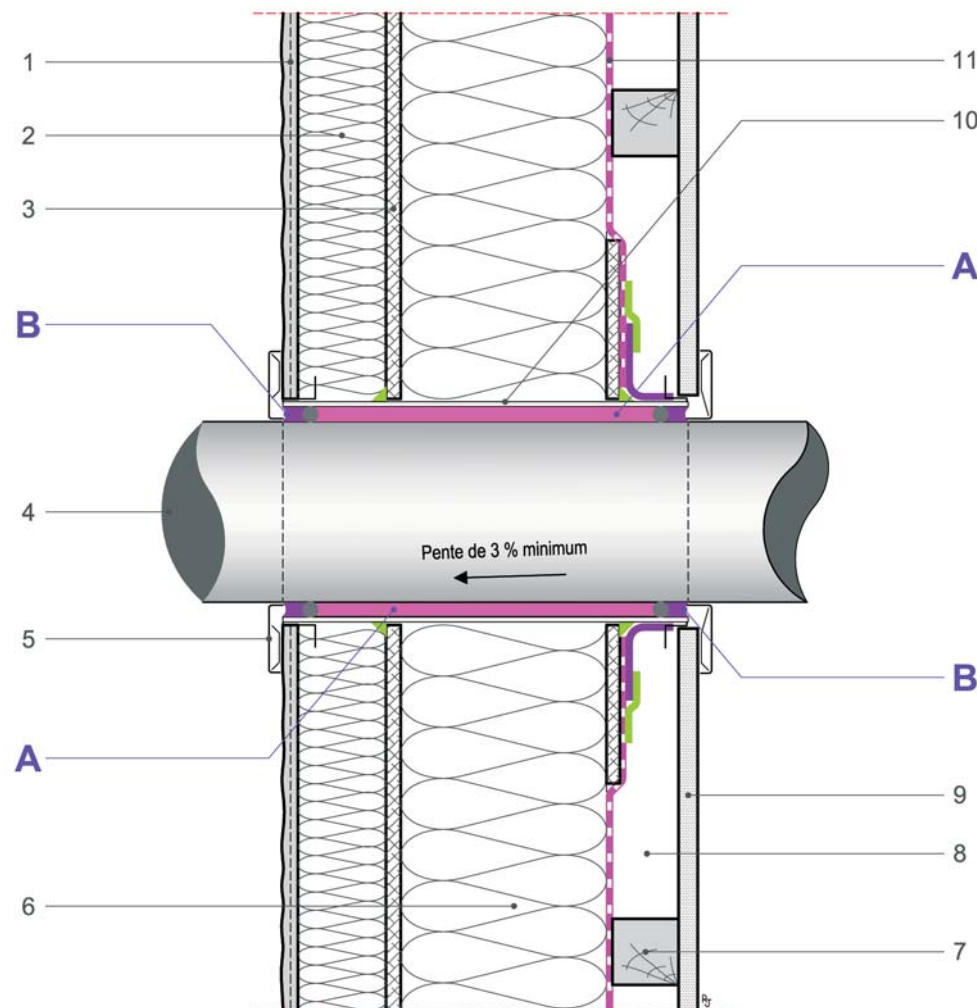
Coupe verticale
