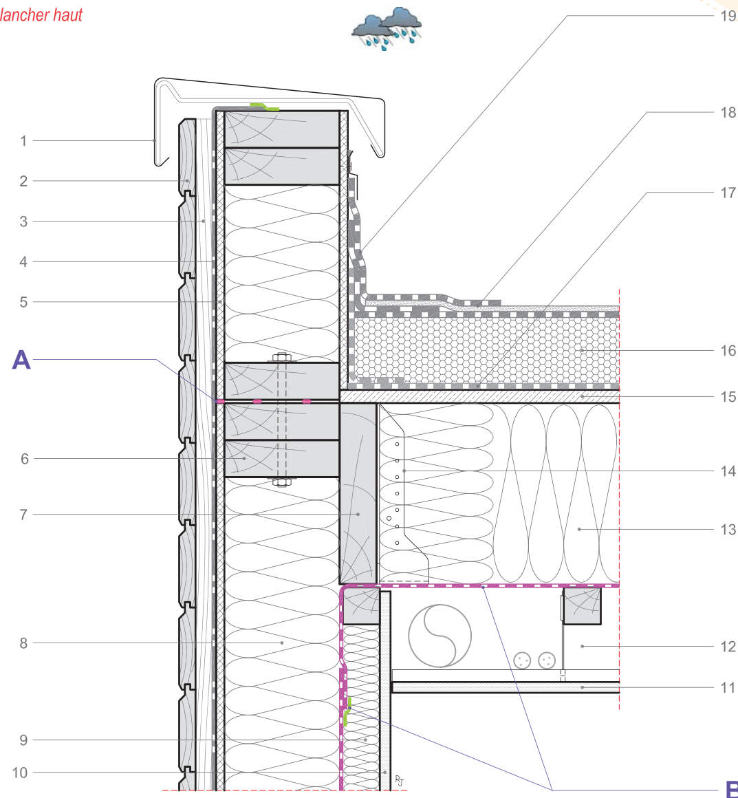
Coupe verticale
