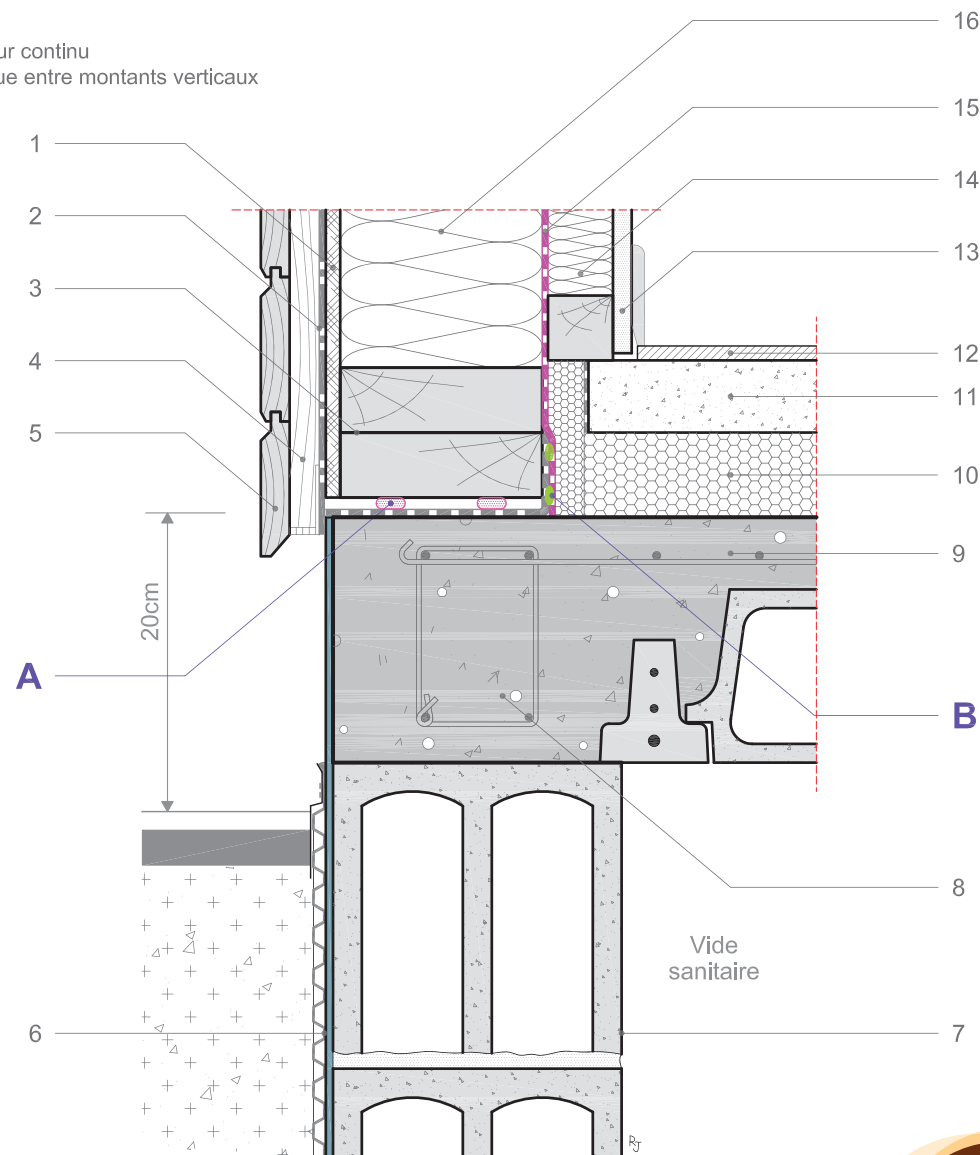
Coupe verticale
