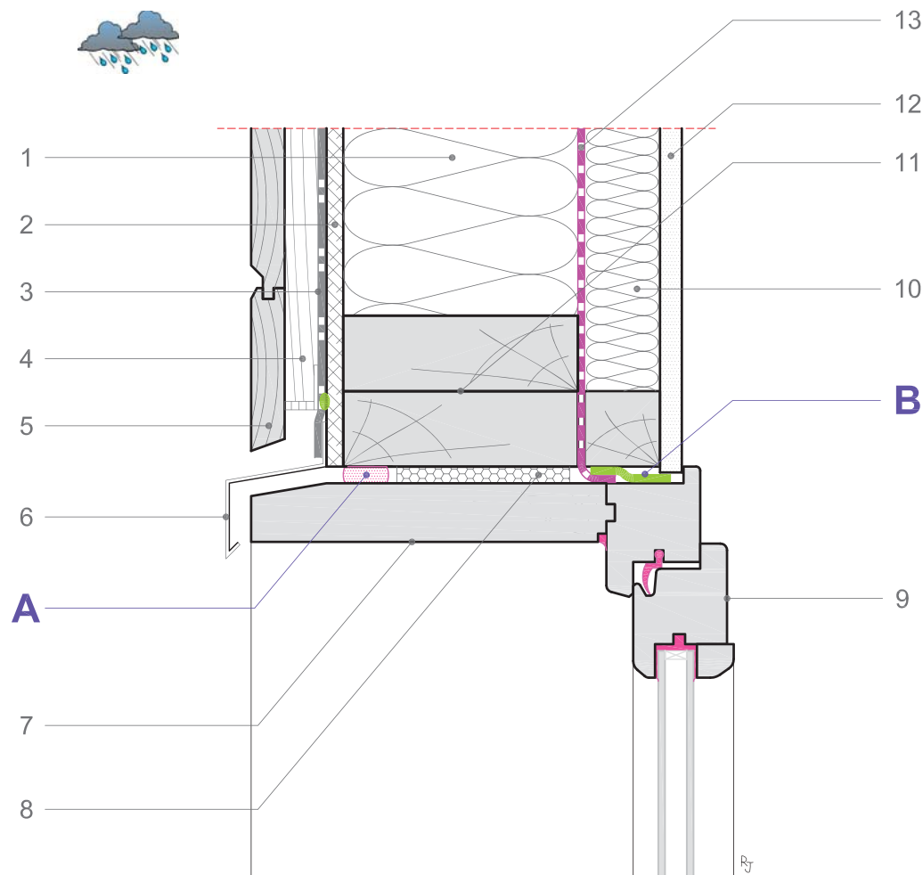
Coupe verticale
