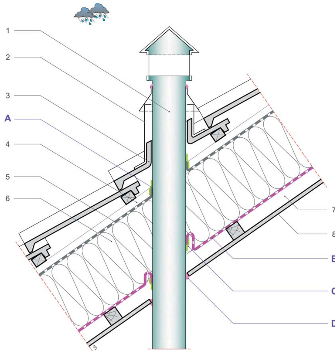
Coupe verticale
