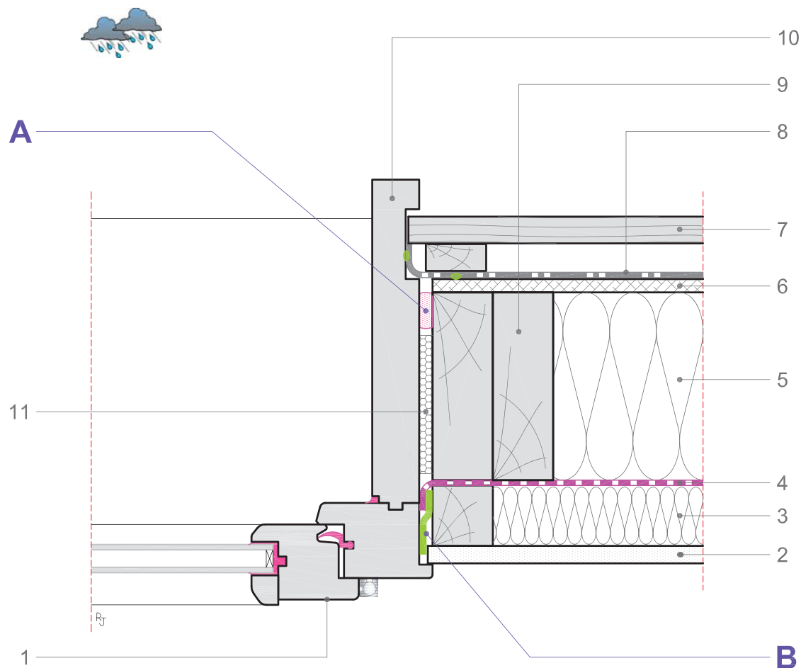
Coupe horizontale
