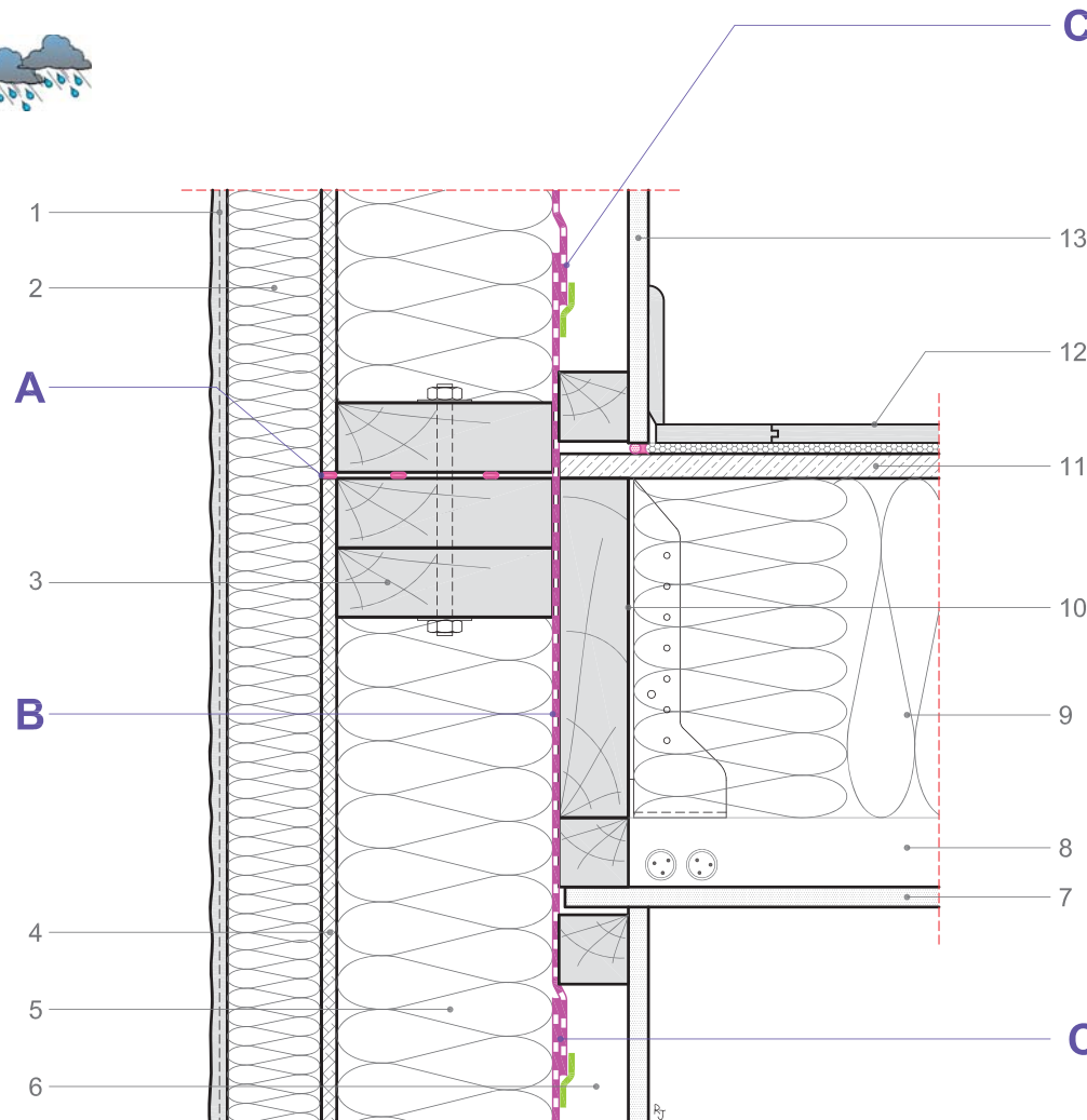
Coupe verticale
