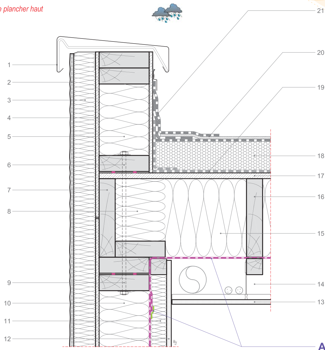
Coupe verticale
