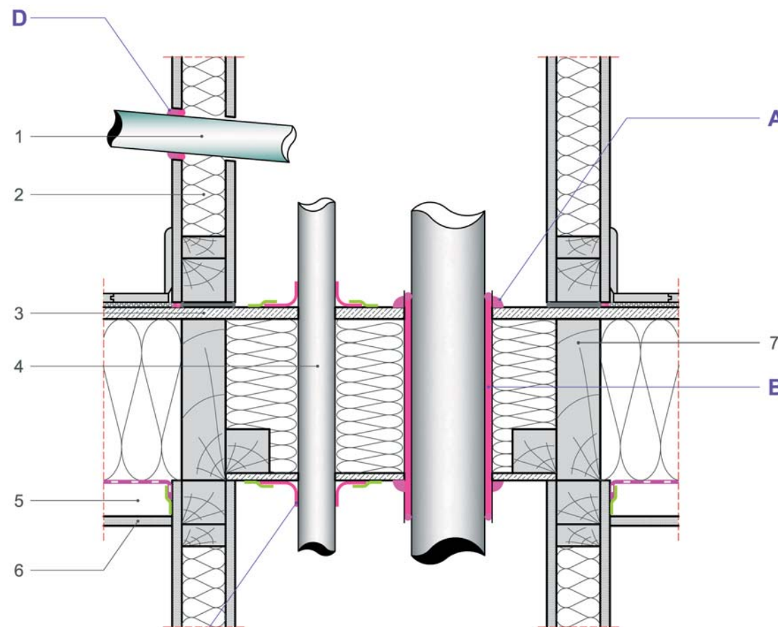
Coupe verticale
