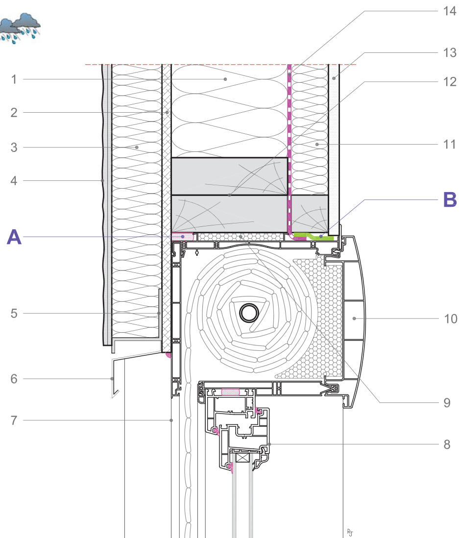
Coupe verticale
