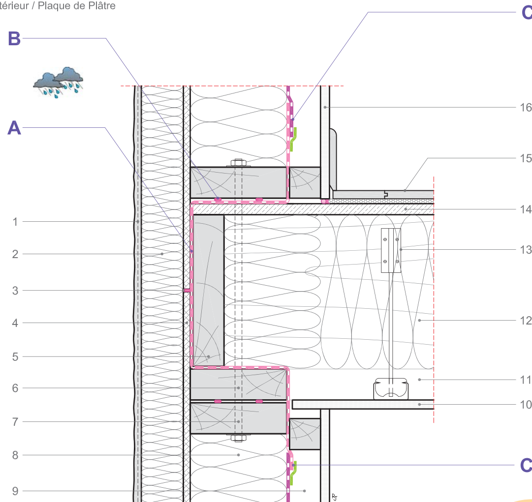
Coupe verticale
