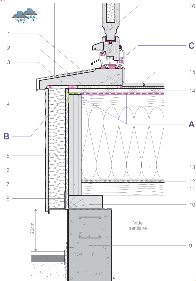
Coupe verticale
