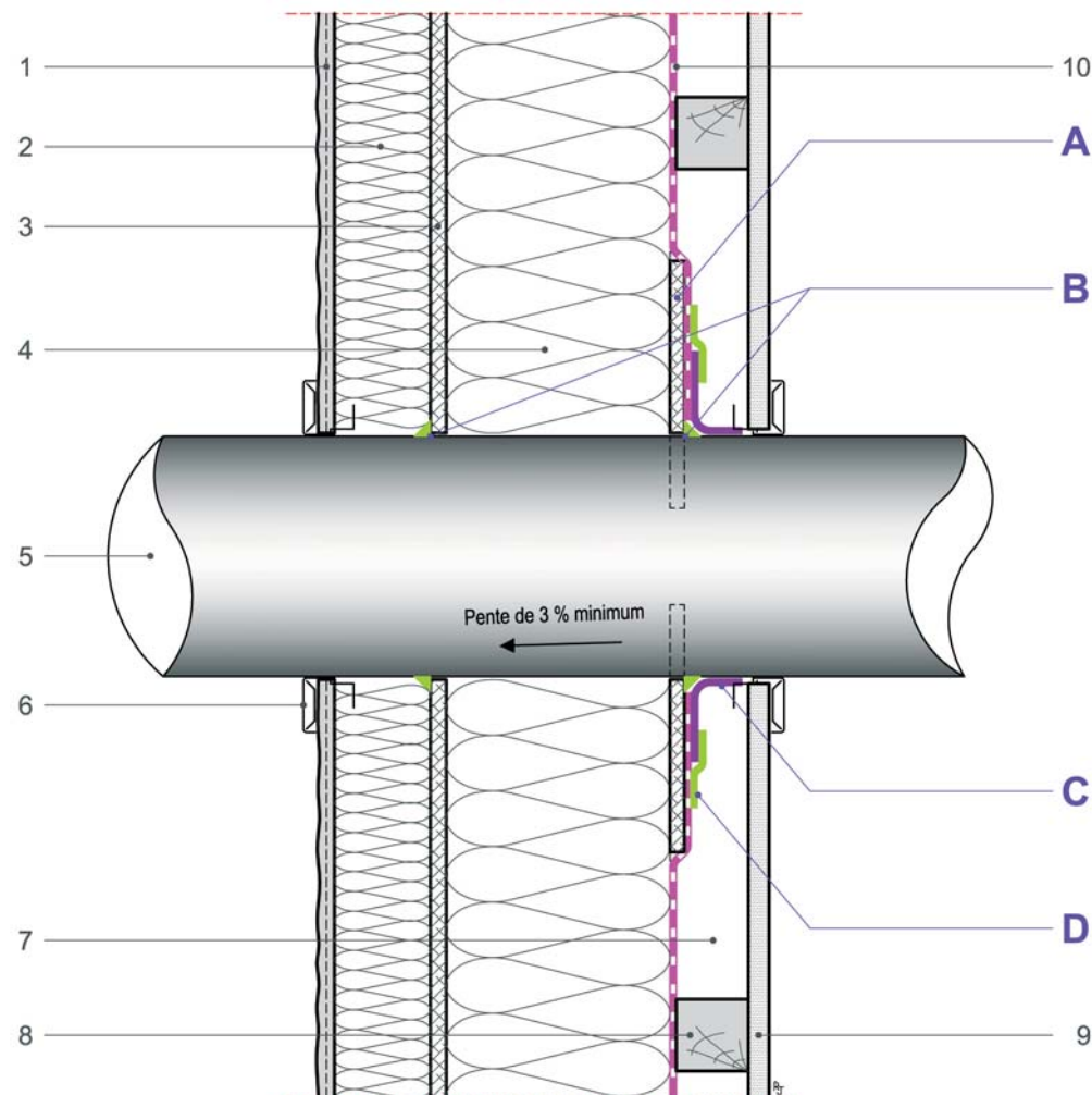
Coupe verticale
