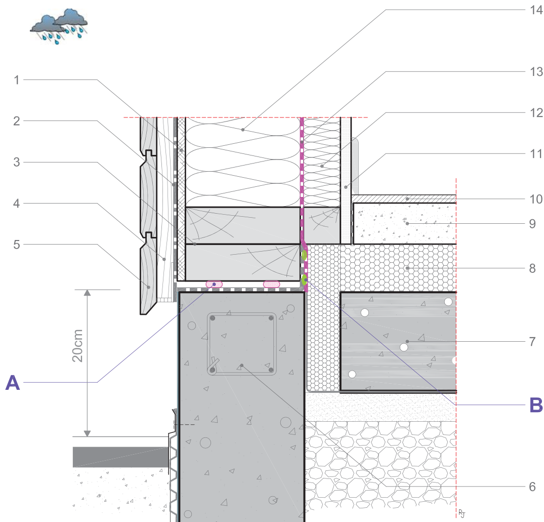
Coupe verticale
