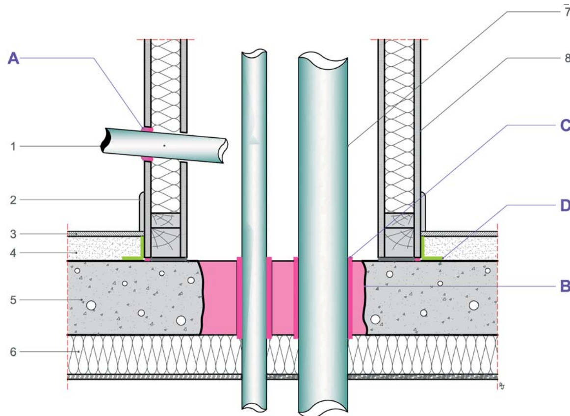
Coupe verticale
