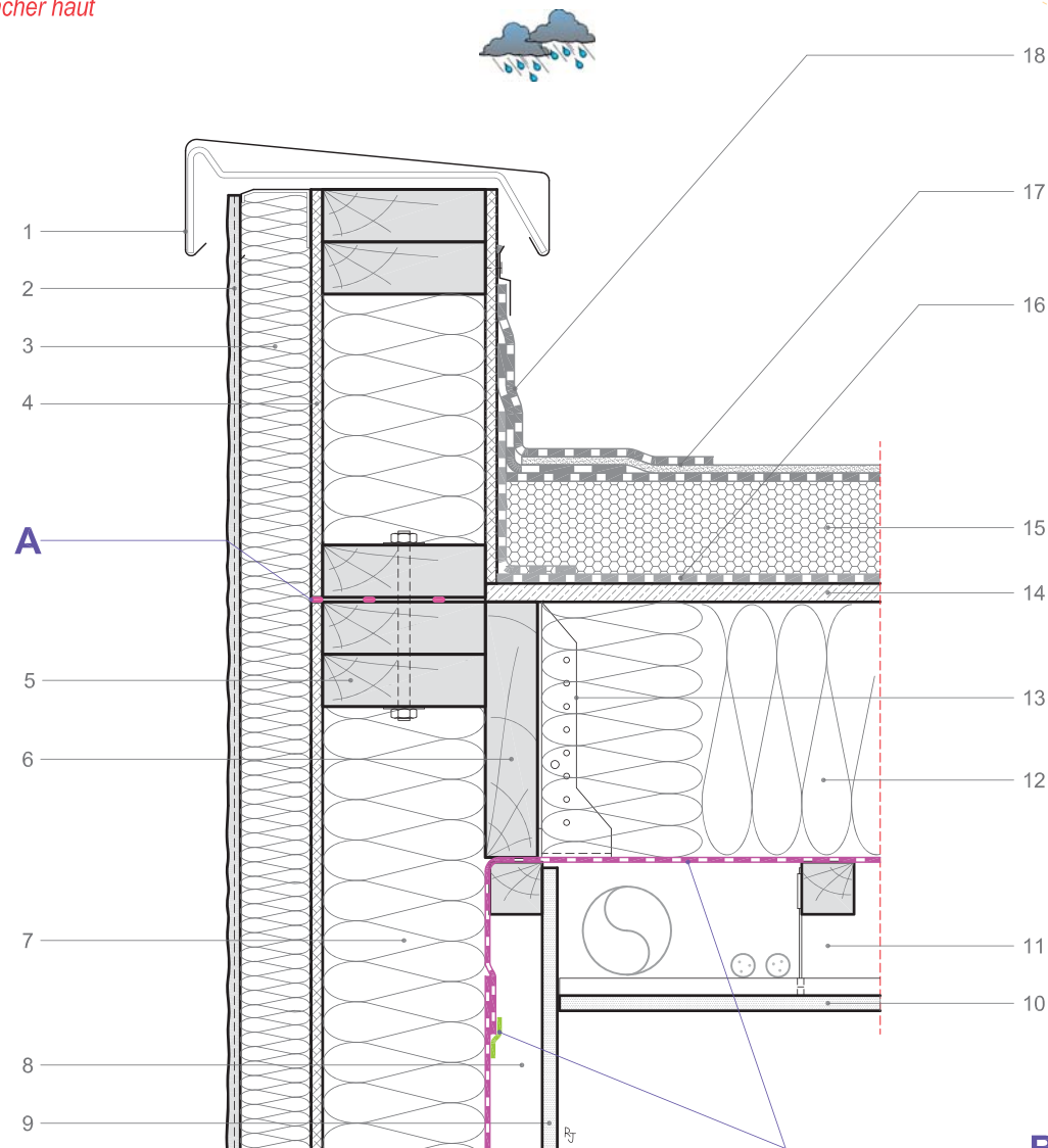
Coupe verticale
