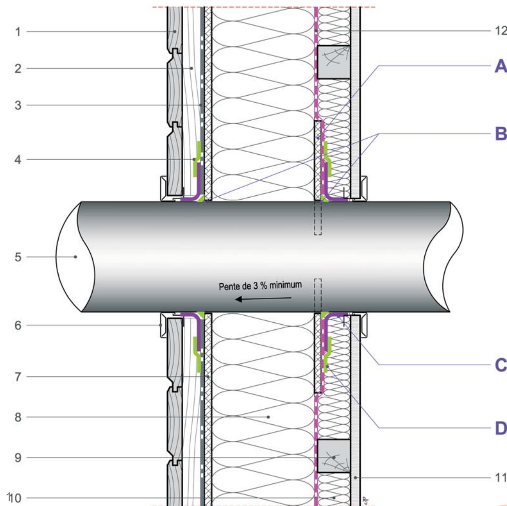
Coupe verticale
