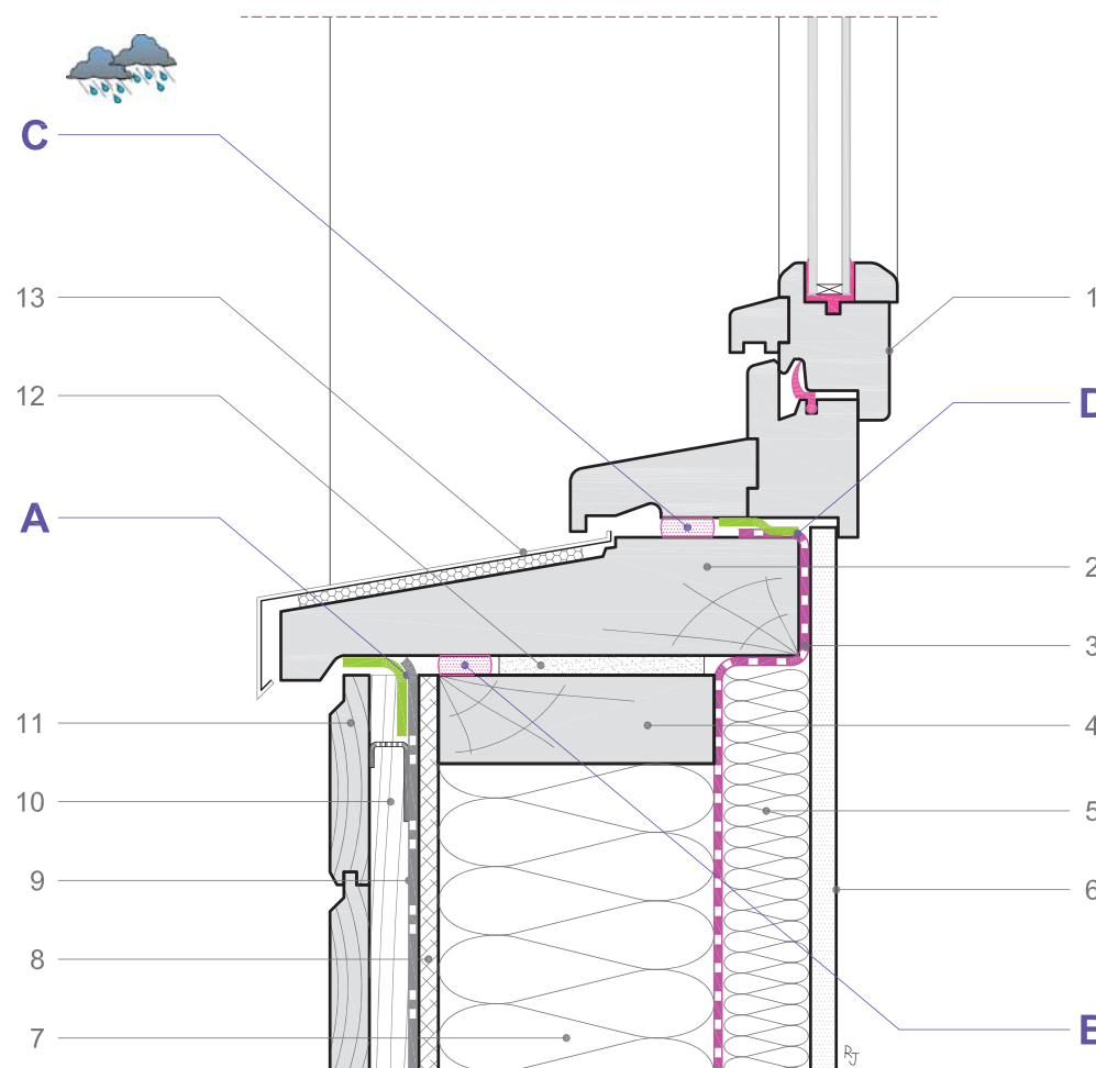
Coupe verticale
