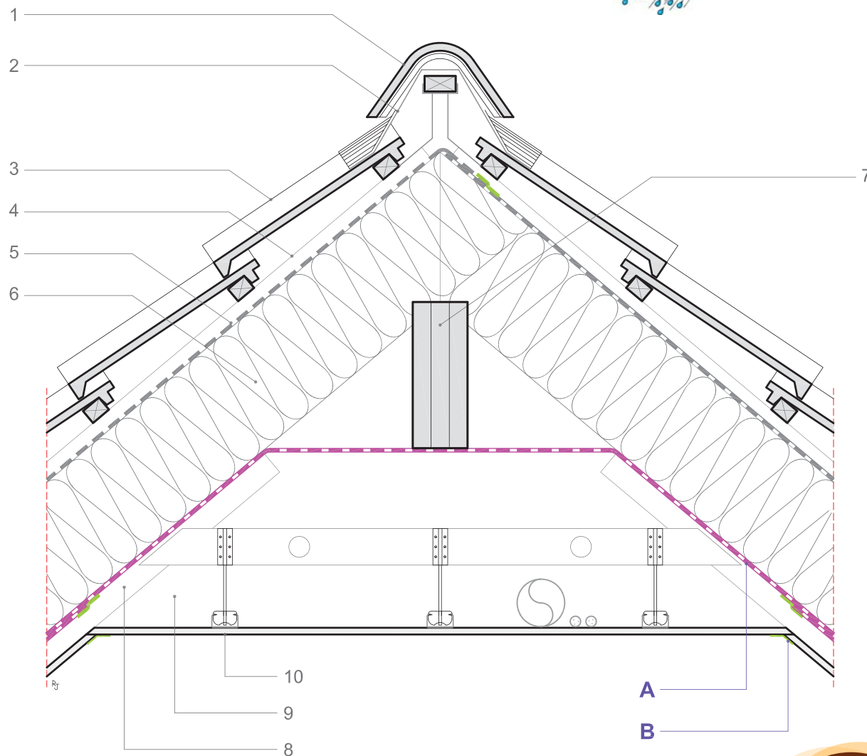
Coupe verticale
