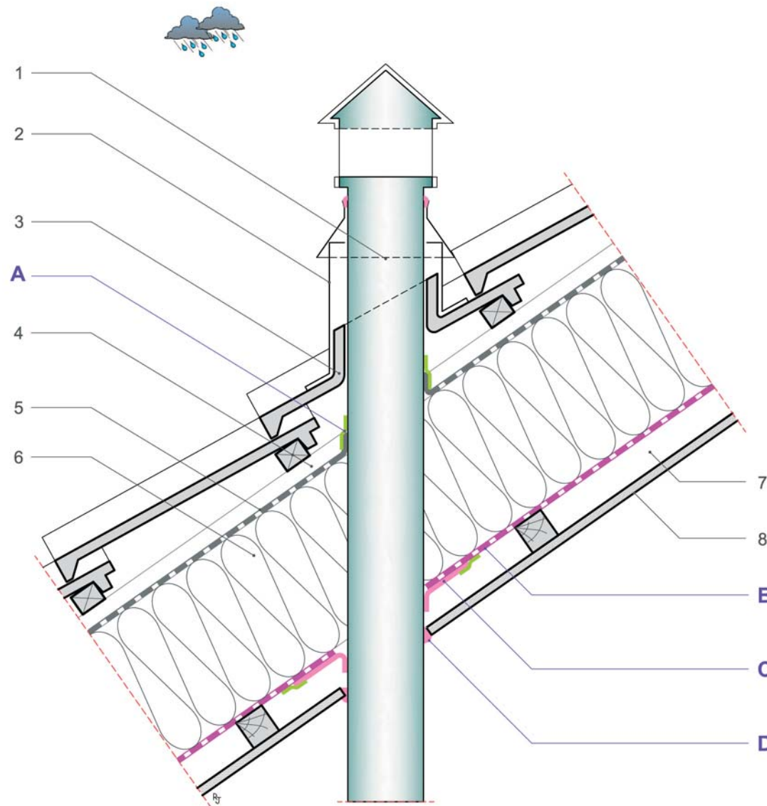
Coupe verticale
