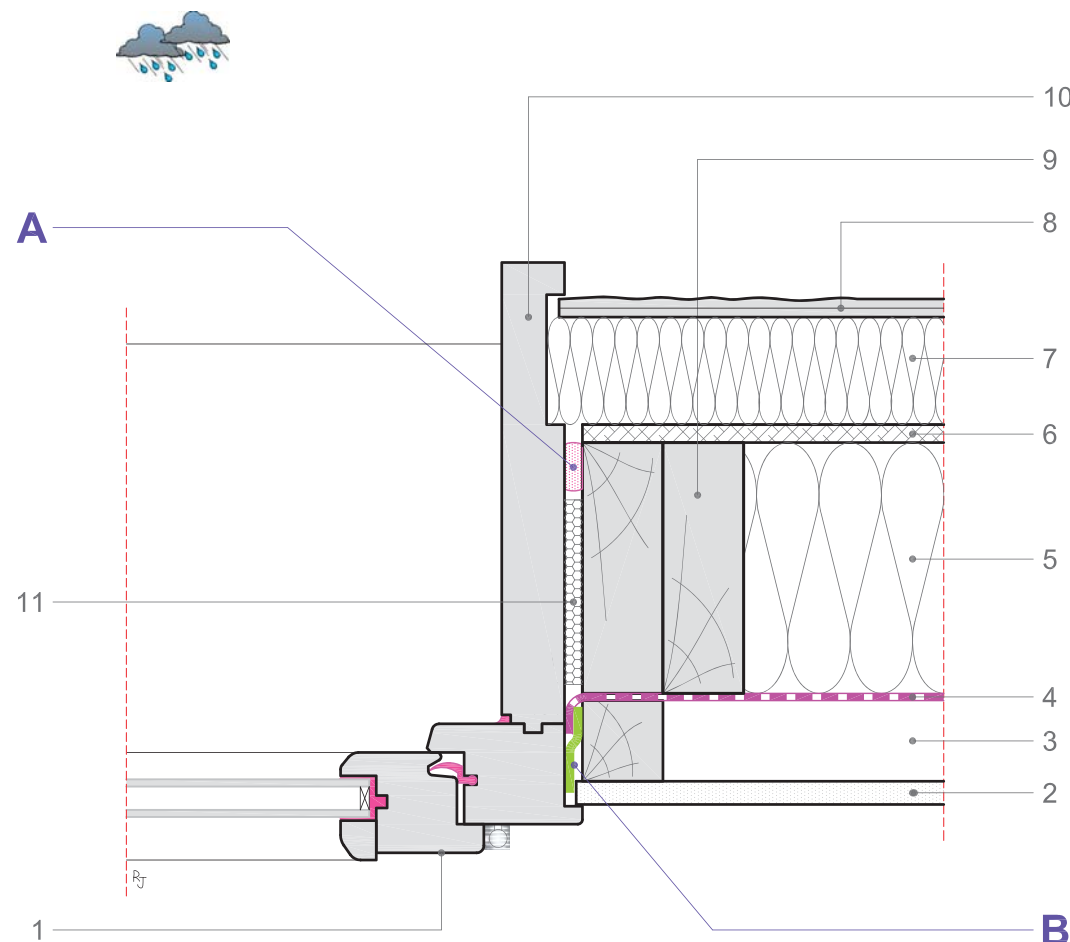
Coupe horizontale
