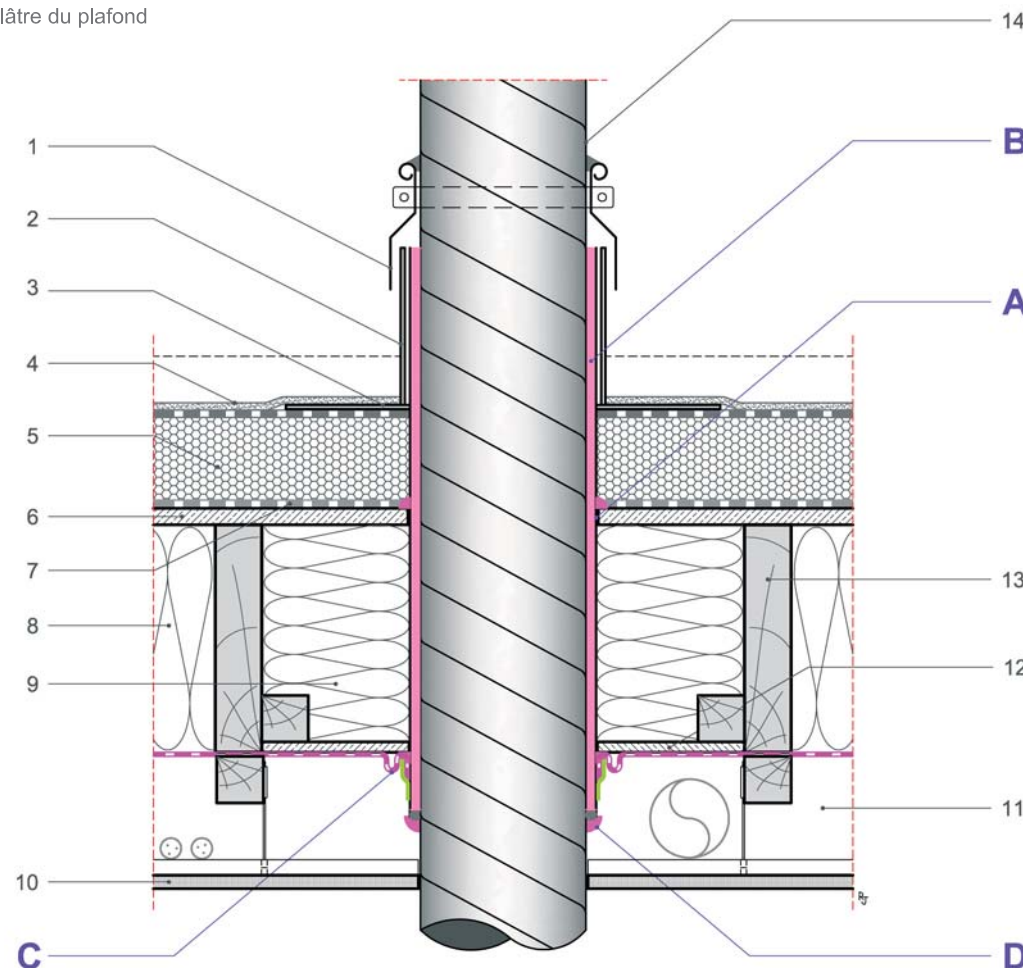
Coupe verticale
