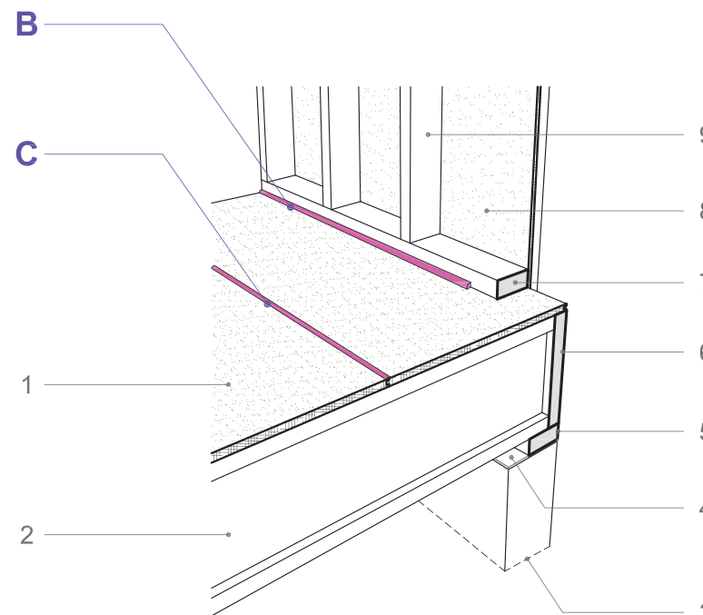
Elévation 3D
