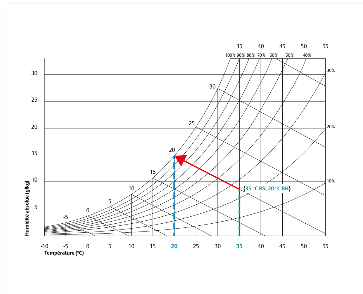
Figure 6. Diagramme psychrométrique
