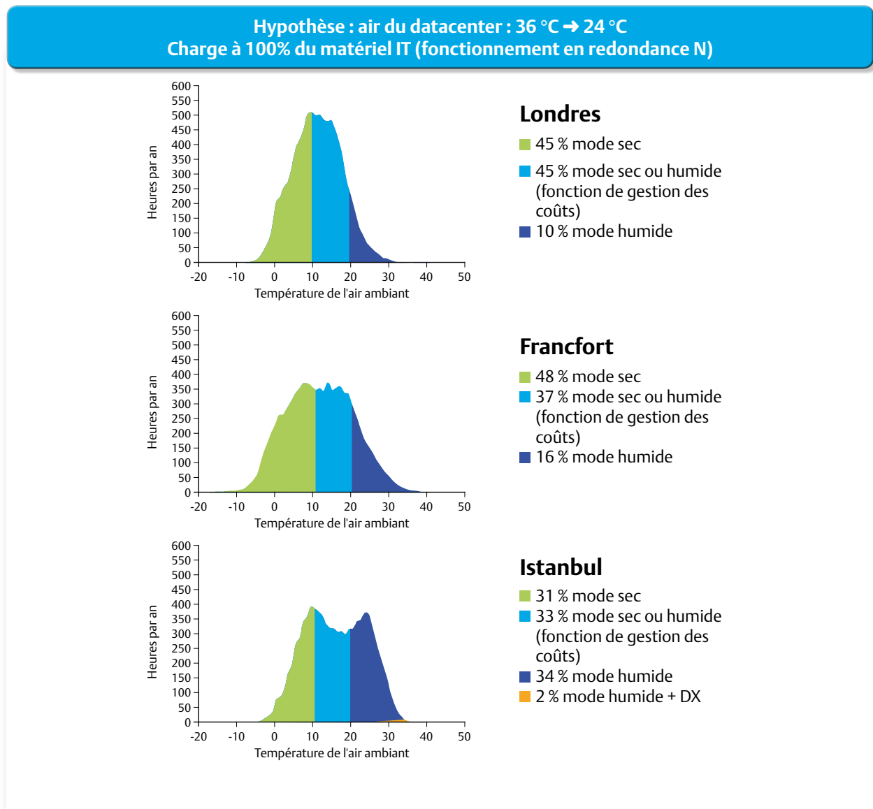
Figure 8. Modes de fonctionnement du groupe Liebert® EFC dans différentes villes
