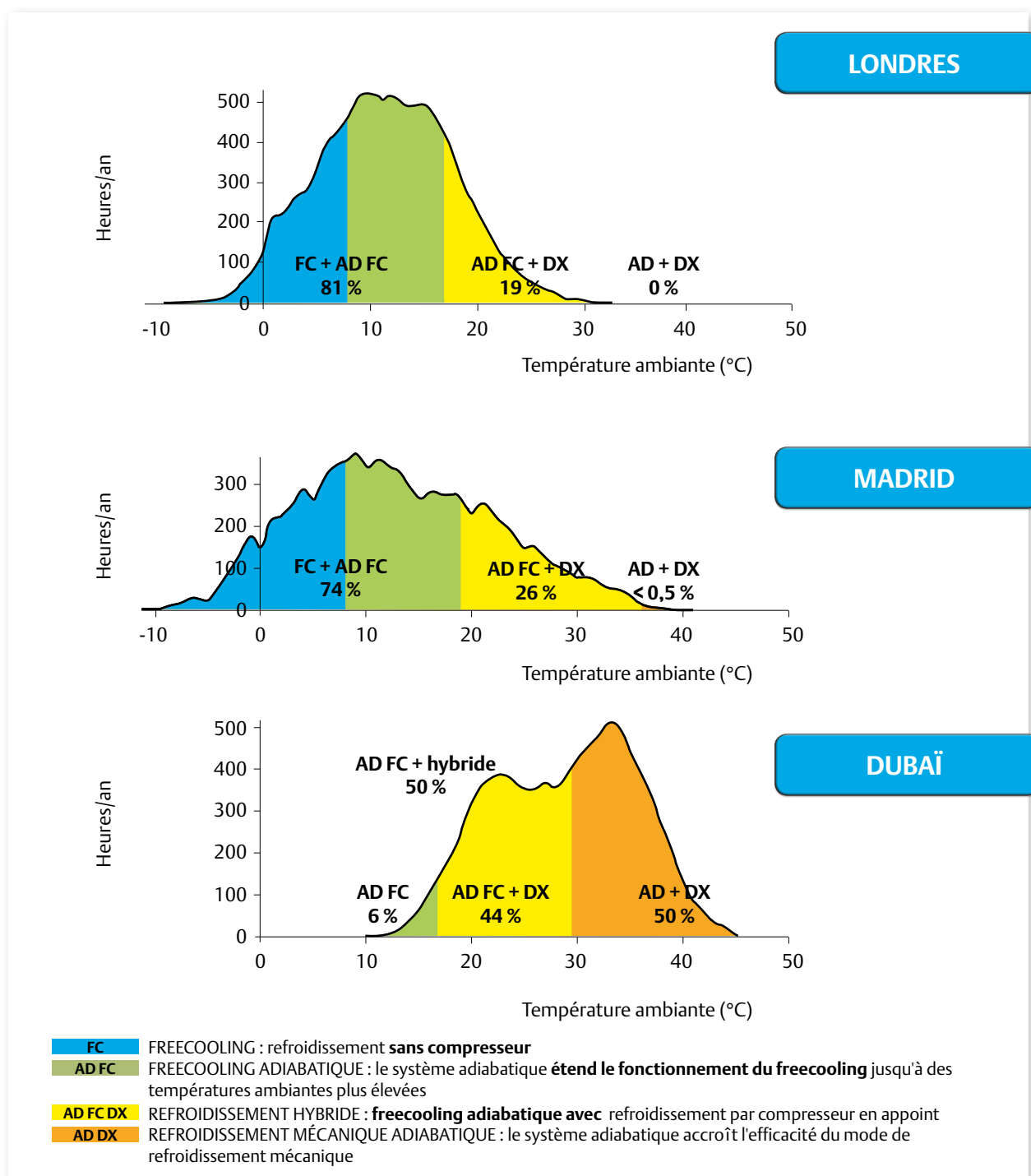
Figure 4. Modes de fonctionnement annuels du système Liebert® AFC à Londres, Madrid, Dubaï, dans un datacenter Tier 4 de 1 MW à pleine charge (groupes d'eau glacée à 50 % de charge) – Mode adiabatique activé pour températures ambiantes > 8 °C
