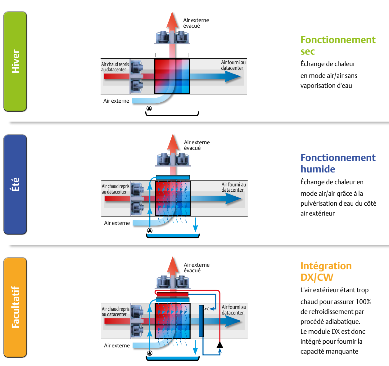
Figure 7. Modes de fonctionnement du groupe Liebert® EFC
