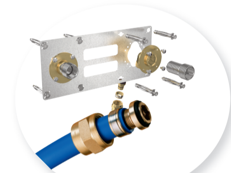
Raccords et tube PER
