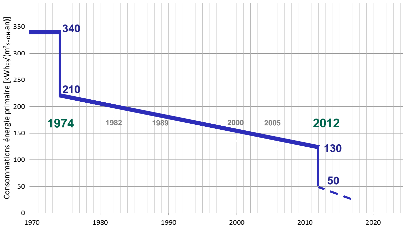
Évolution des consommations réglementaires 5 usages en kWh EP /(m 2 .an) pour bâtiments résidentiels avec combustibles en zone H2
