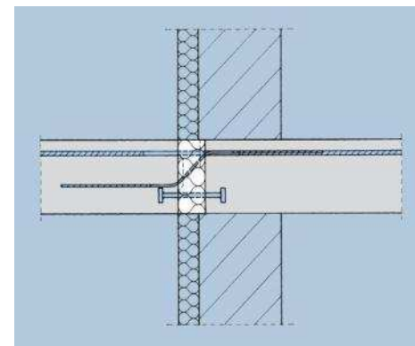
Rutec PLAKABETON ( \Psi \approx 0.26 )
